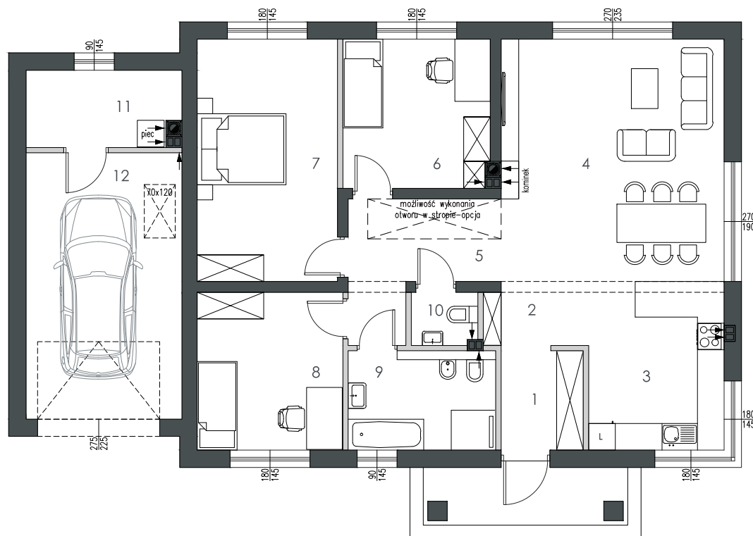
rzut parteru
